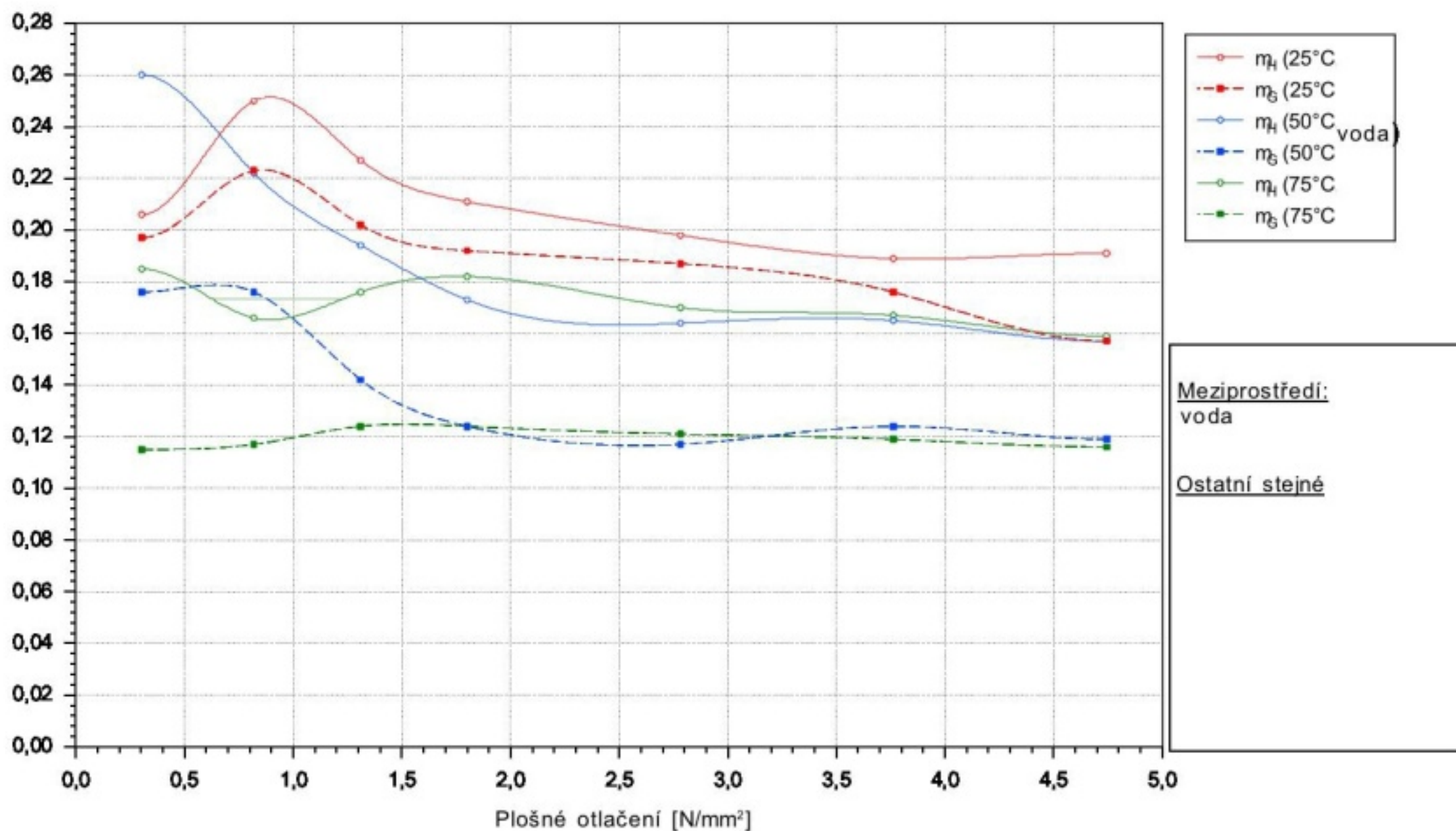
Obr. 71 Hodnota tření ZX-530 při mazání vodou; měřená po záběhu
