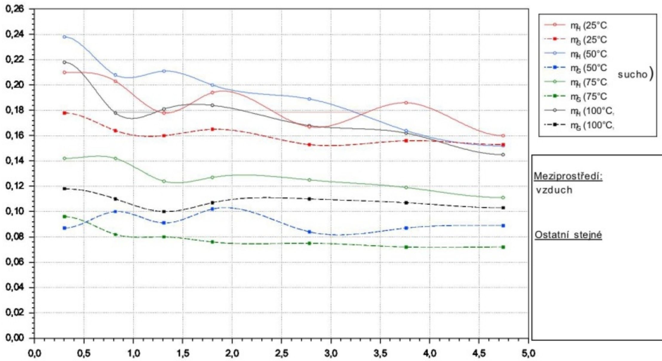
Obr. 70 Hodnota tření ZX-530 při chodu za sucha; měřená po záběhu
