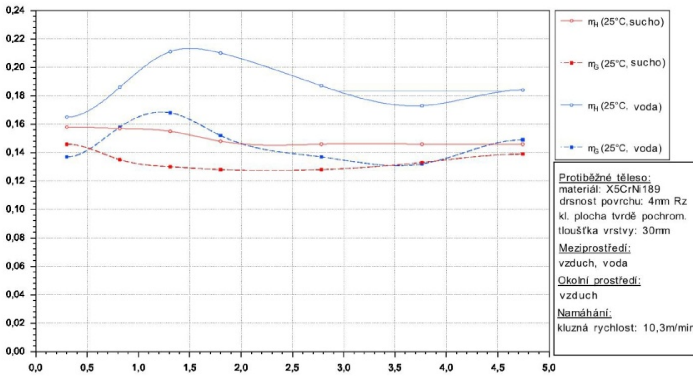
Obr. 69 Hodnota tření ZX-530; měřená v dodávaném stavu
